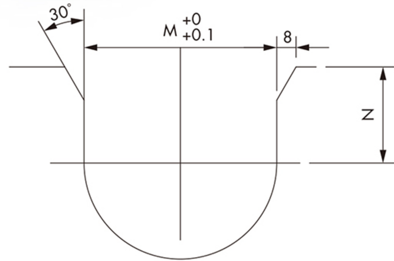
模具定位孔尺寸 Mold position hole size
